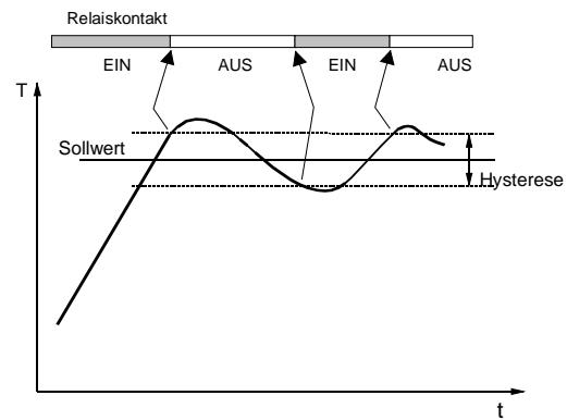
Bild 2: Heizregler, symmetrische Hysterese
