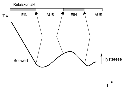
Bild 3: Kühlregler, einseitige Hysterese
