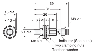
Fig. 29: E2E-X4MD□-M3G/E2E-X2ME□-M3/F□-M3
