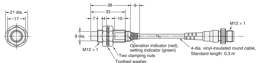
Fig. 32: E2E-X7D1-M1GJ E2E-X7D1-M1J-T
