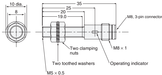
Fig. 37: E2E-X1□□-M5
