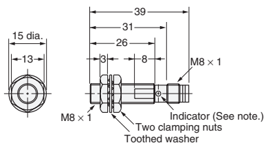
Fig. 28: E2E-X2D□-M3G/E2E-X1R5E□-M3/F□-M3
