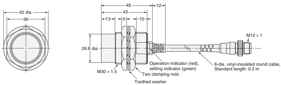
Fig. 35: E2E-X20MD1-M1GJ
